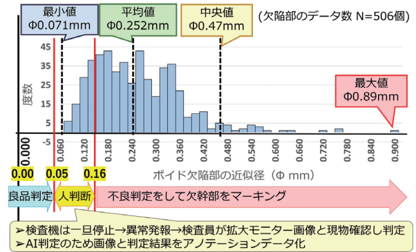
図3 欠陥部の画像処理検査判定方法
