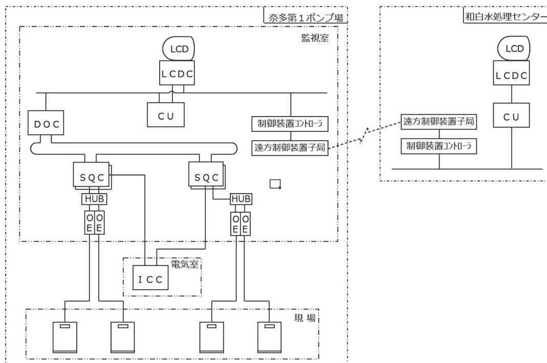
図5 システム構成図
