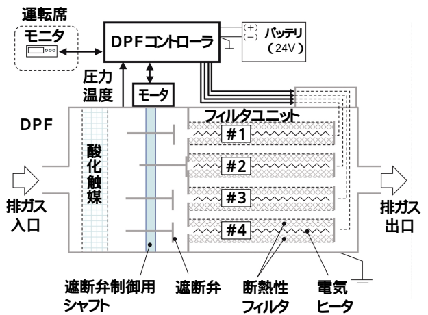
図2 電気ヒータ再生式DPFシステムの模式図
