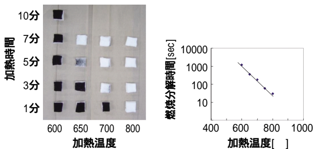
図1 ディーゼル排ガス中のカーボン粒子の酸化燃焼特性
